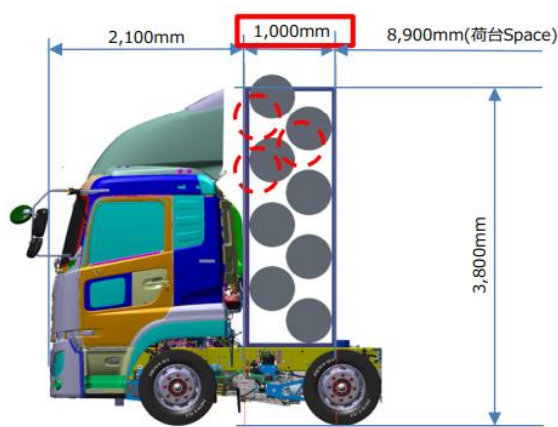
《図表 5》FCV 化に伴う荷台スペース減少イメージ
