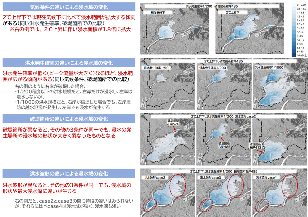
図表3 気候条件、洪水発生確率、破堤箇所、洪水波形の違いによる浸水域の変化
