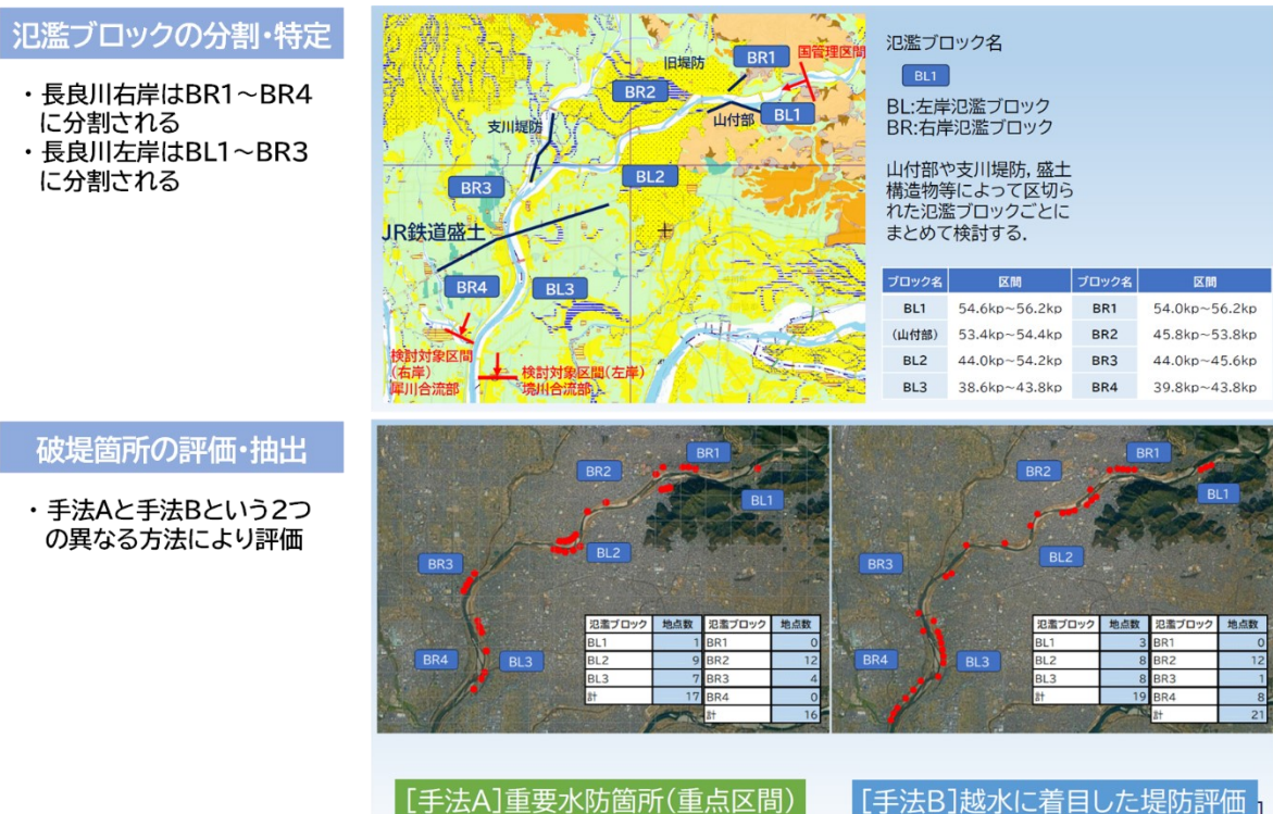
図表2 氾濫ブロックの分割・特定と破堤点の評価・抽出
