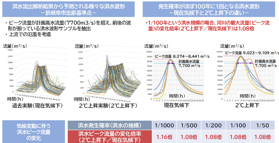
図表1 気候変動に伴う洪水波形や洪水ピーク流量の変化
