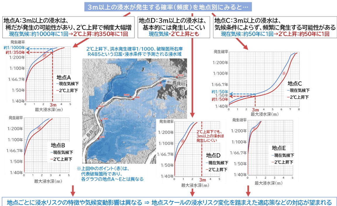
図表9 気候変動に伴う地点スケールの浸水リスク変化(25m メッシュごとの浸水発生確率カーブ)
