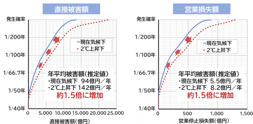
図表8 気候変動に伴う地域スケールの水害リスク変化（被害発生確率カーブの例）
